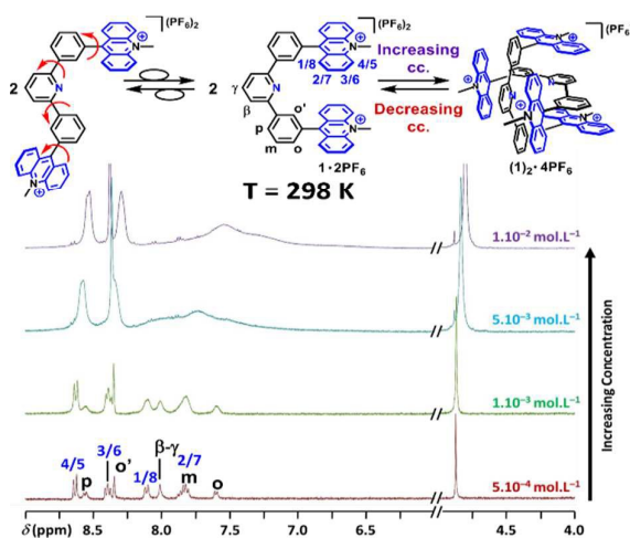
Fig. 1 ^1\text{H} NMR (500 MHz, \text{CD}_3\text{CN} , 298 K) spectra of 1·2PF 6 at 1 \cdot 10^{-2} , 5 \cdot 10^{-3} , 1 \cdot 10^{-3} and 5 \cdot 10^{-4} \text{ mol} \cdot \text{L}^{-1} .
